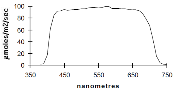
SKP215 分光感度特性
